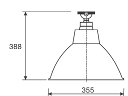
Lamp: E40 175W max
