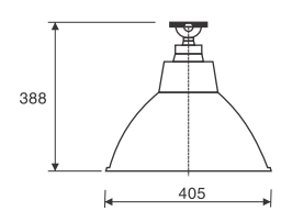
Lamp: E40 250W max
